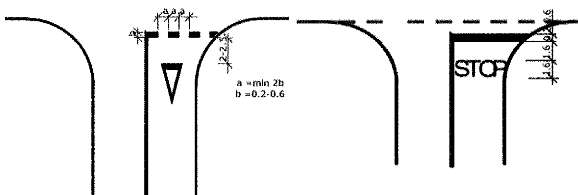
Fig. 6. Vija gjatësore e plote e mesit dhe vijat tërthore të ndërprera dhe plota (vija STOP).
