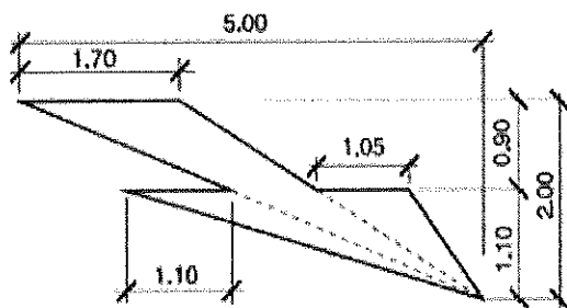
Figura. 10. Dimensionet e shigjetave dhe forma e ekzekutimit.
