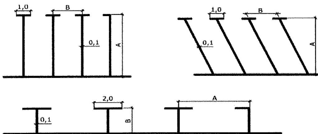
Figura 4. Vija gjatësore e ndërprerë dhe e plotë e parkingjeve.
