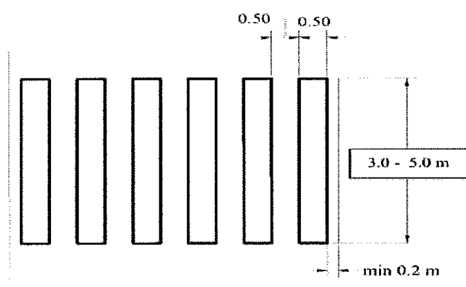
Figura .5. Vendkalimi i këmbësorëve përcakton pjesën e rrugës të destinuar për kalim e këmbësorëve dhe dimensionet.
