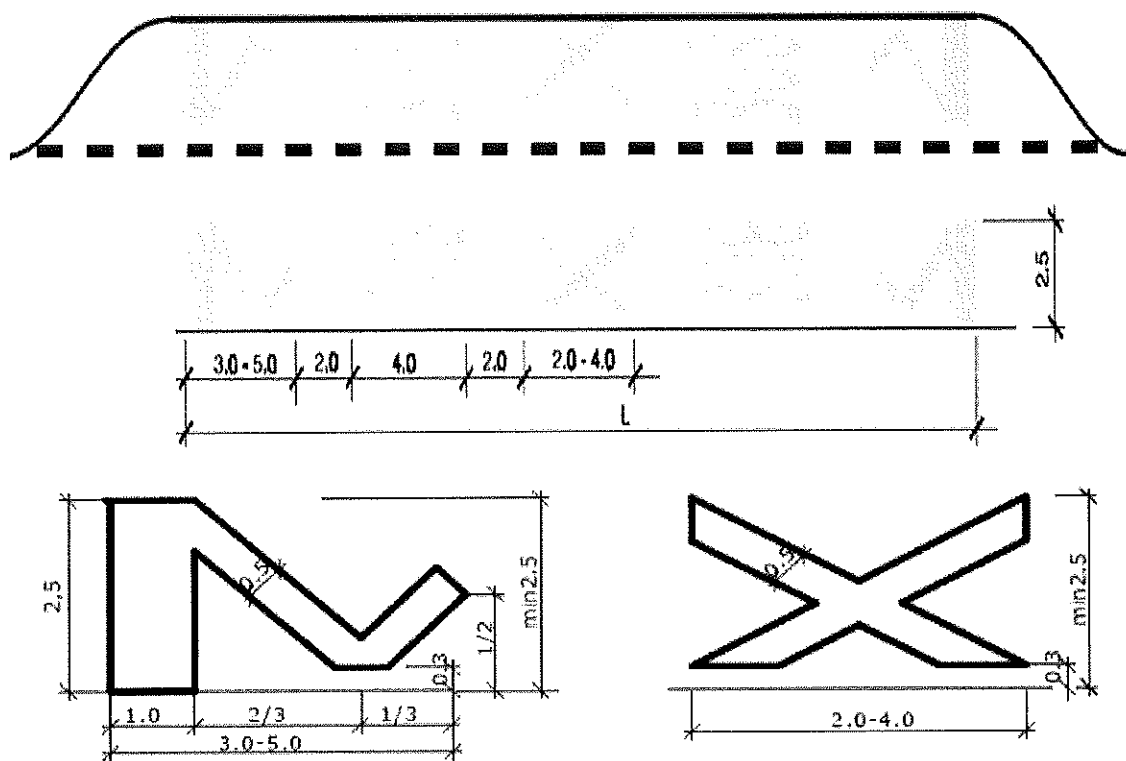
Figura 9. Shënimi i sipërfaqeve të trafikut për nevojat të veçanta shërbim
